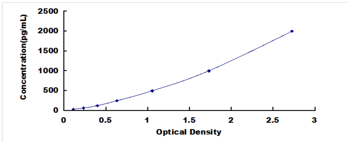
大鼠多配体蛋白聚糖 4 (SDC4) 检测试剂盒标准曲线
