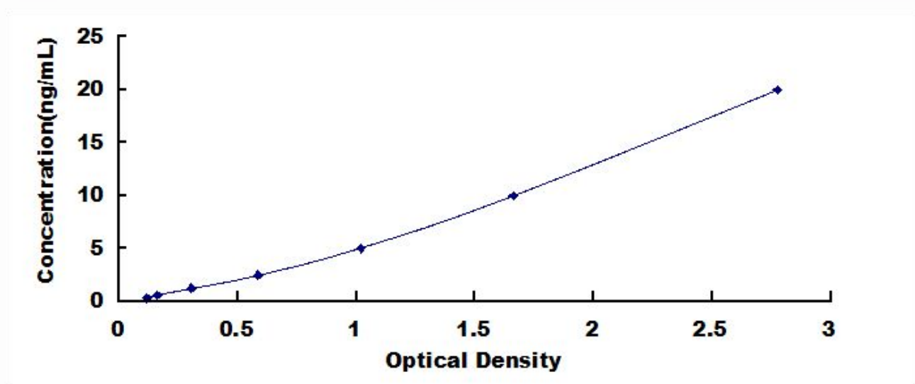
人 Ig 和 ITIM 域蛋白 T-细胞免疫受体 (TIGIT) 检测试剂盒标准曲线
