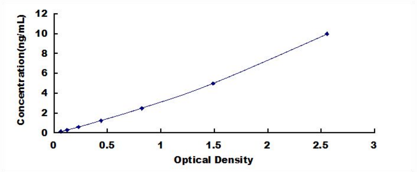
人硫氧还蛋白结合蛋白 2 (TBP2) 检测试剂盒标准曲线
