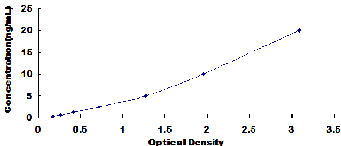
人硫氧还蛋白还原酶 1(TrxR1)检测试剂盒标准曲线
