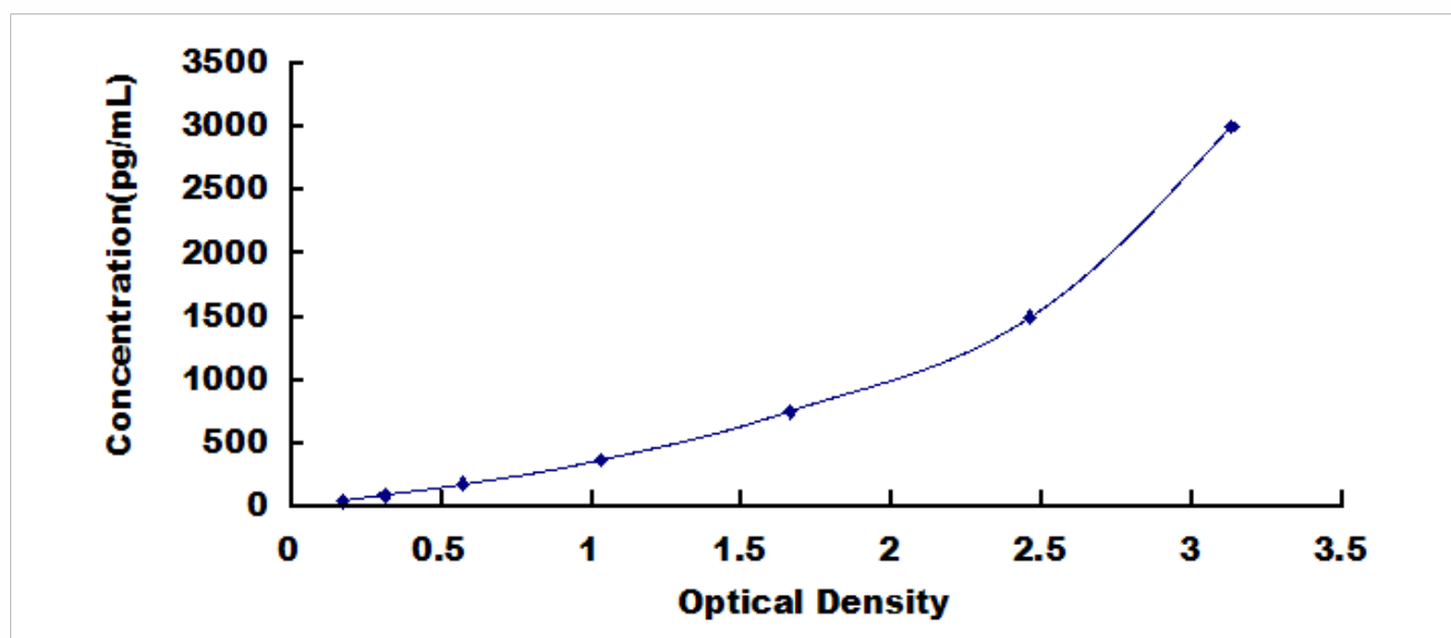
人血栓调节蛋白(TM)检测试剂盒标准曲线
