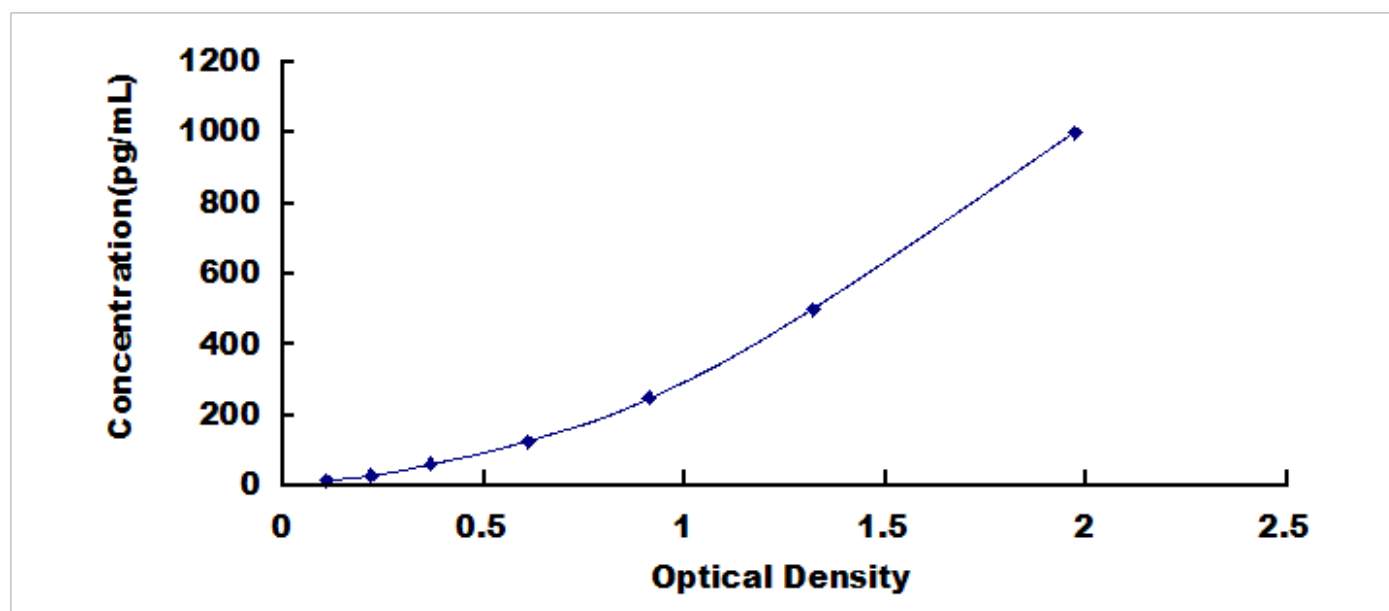
大鼠血小板生成素(TPO)检测试剂盒标准曲线
