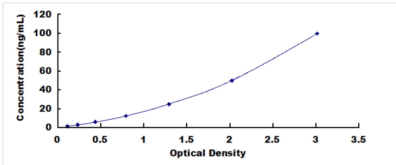
人血小板反应蛋白 3 (THBS3) 检测试剂盒标准曲线
