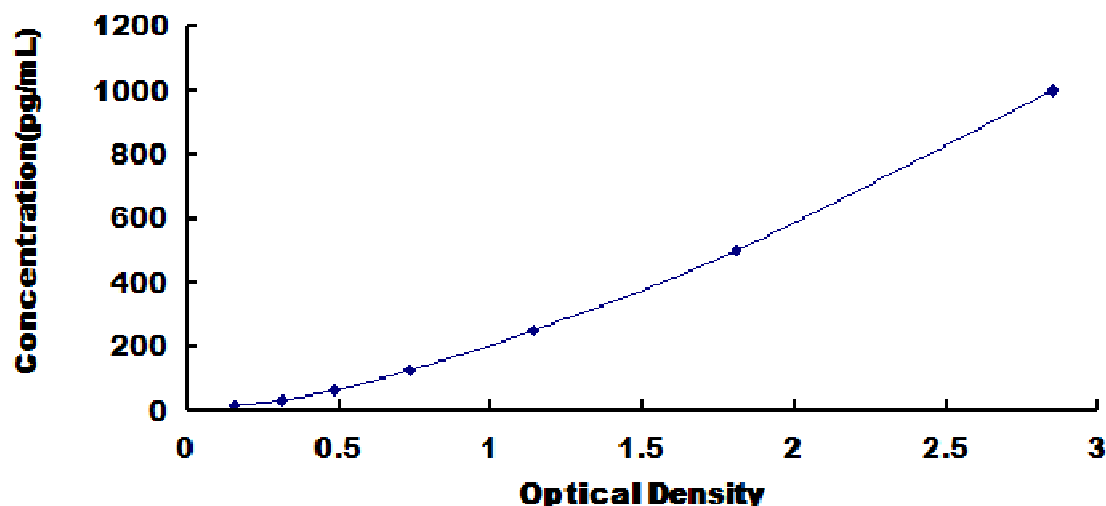
人可溶性胸苷激酶 1 (TK1) 检测试剂盒标准曲线
