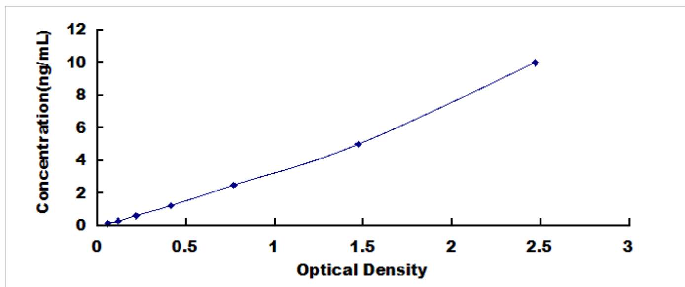
人胸腺嘧啶核苷磷酸化酶(TP)检测试剂盒标准曲线
