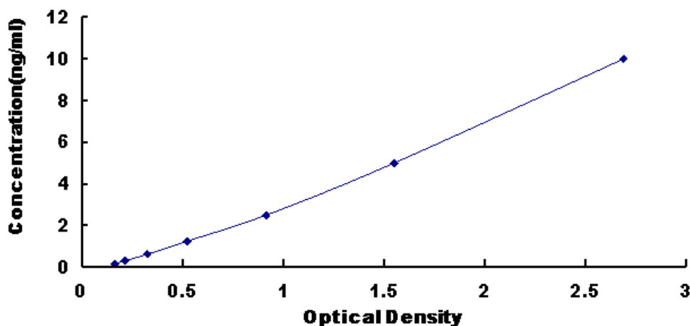
图 1：人的拓扑异构酶 I(TOP1)试剂盒标准曲线
