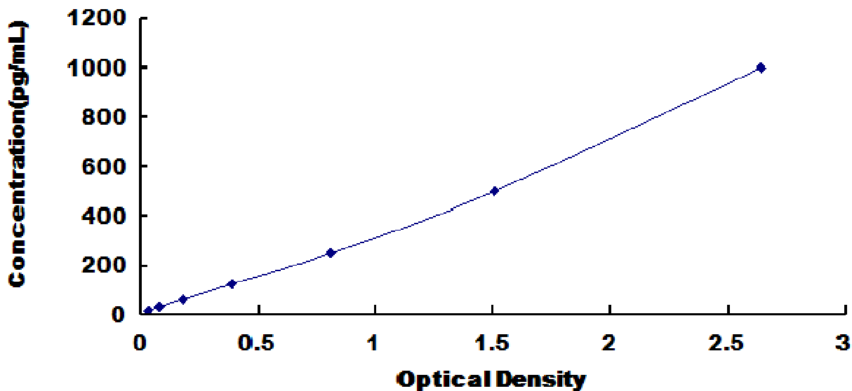
人转化生长因子 \alpha (TGF \alpha )检测试剂盒标准曲线
