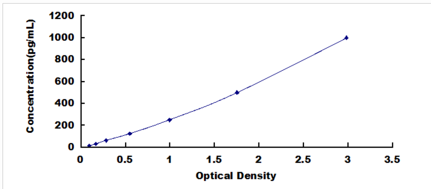
小鼠转化生长因子 \beta 1 (TGF \beta 1) 检测试剂盒标准曲线
