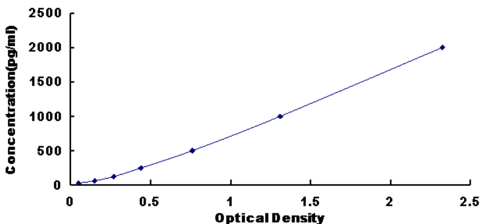
图 1: 牛的转化生长因子 \beta 2(TGF \beta 2)试剂盒标准曲线
