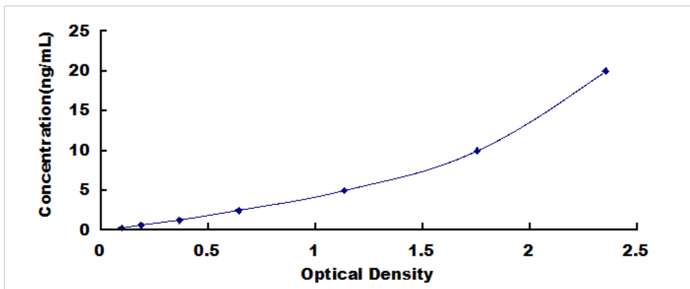
人转化生长因子β受体II (TGF β R2) 检测试剂盒标准曲线
