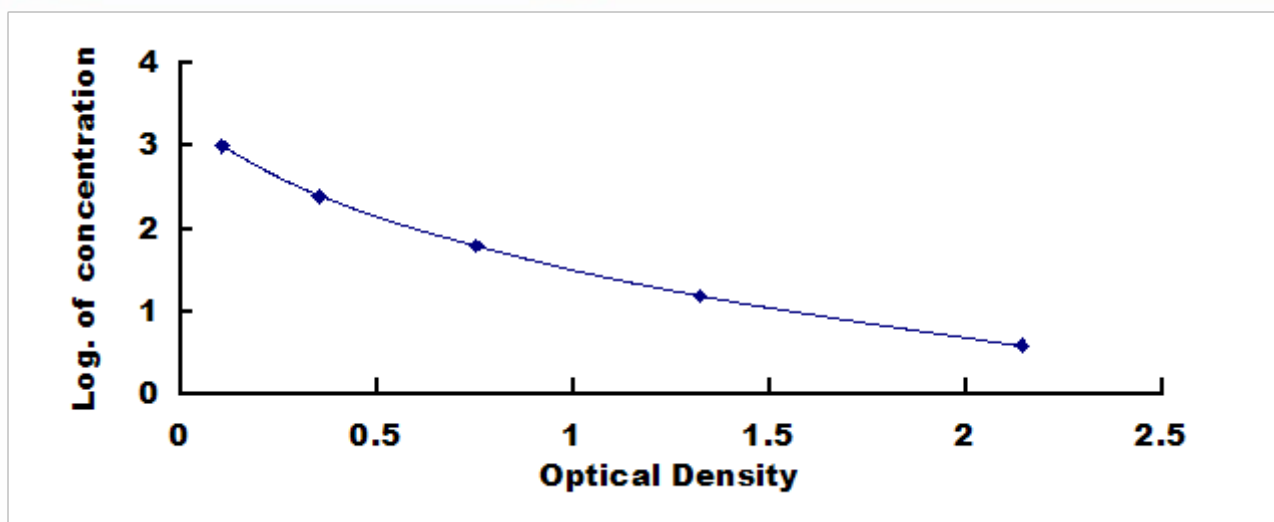
甘油三酯(TG)检测试剂盒标准曲线
