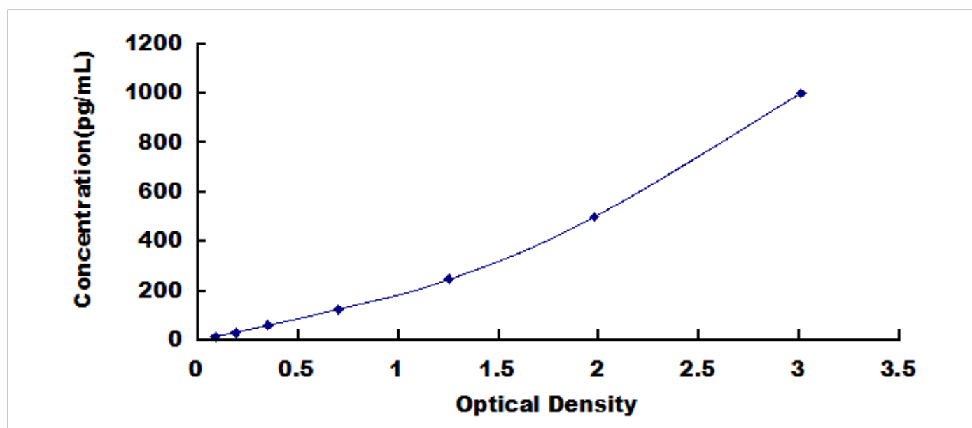
兔心肌肌钙蛋白 I (TNNI3) 检测试剂盒标准曲线
