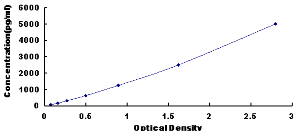
图 1：牛的肿瘤坏死因子 \alpha (TNF \alpha )试剂盒标准曲线
