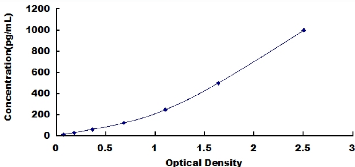
山羊肿瘤坏死因子 \alpha (TNF \alpha ) 检测试剂盒标准曲线
