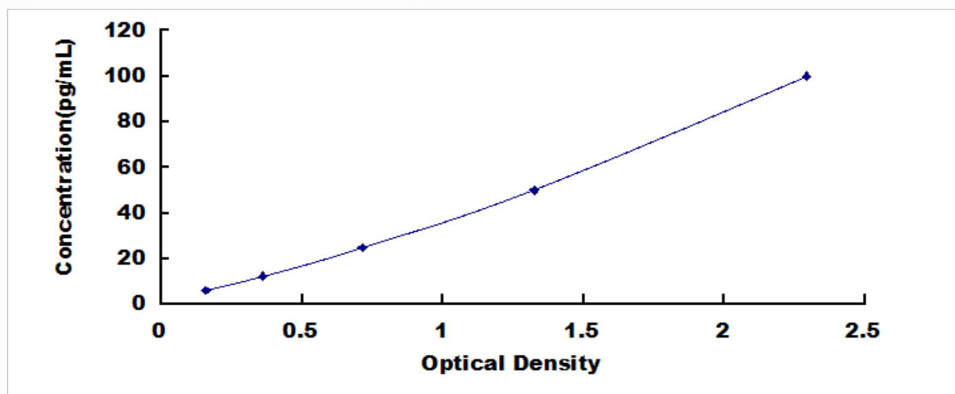
人肿瘤坏死因子 \alpha (TNF \alpha ) 检测试剂盒标准曲线
