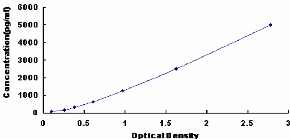
图 1：大鼠肿瘤坏死因子配体超家族成员 12(TNFSF12)试剂盒标准曲线
