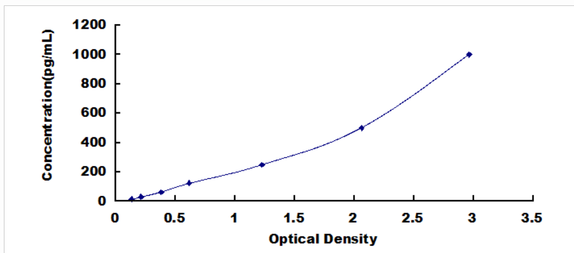
小鼠肿瘤坏死因子相关凋亡诱导配体 (TRAIL) 检测试剂盒标准曲线
