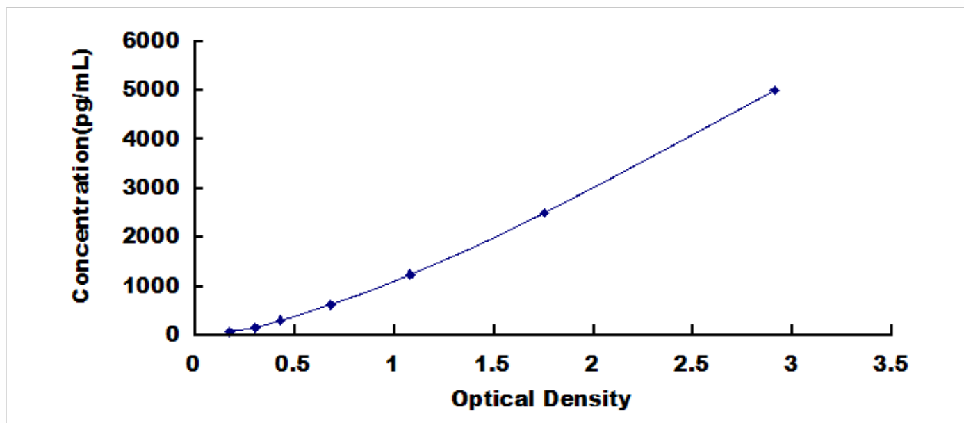
大鼠肿瘤蛋白 p53 (TP53) 检测试剂盒标准曲线
