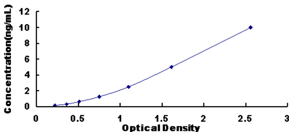
图 1：大鼠酪氨酸羟化酶(TH)试剂盒标准曲线
