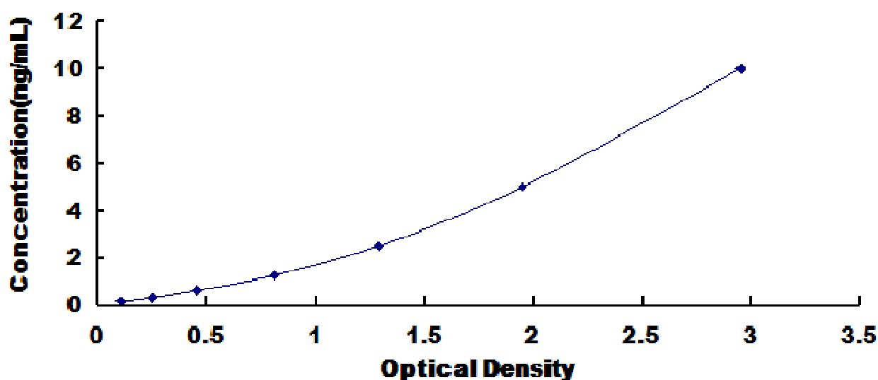
人尿嘧啶 DNA 糖基化酶(UNG)检测试剂盒标准曲线
