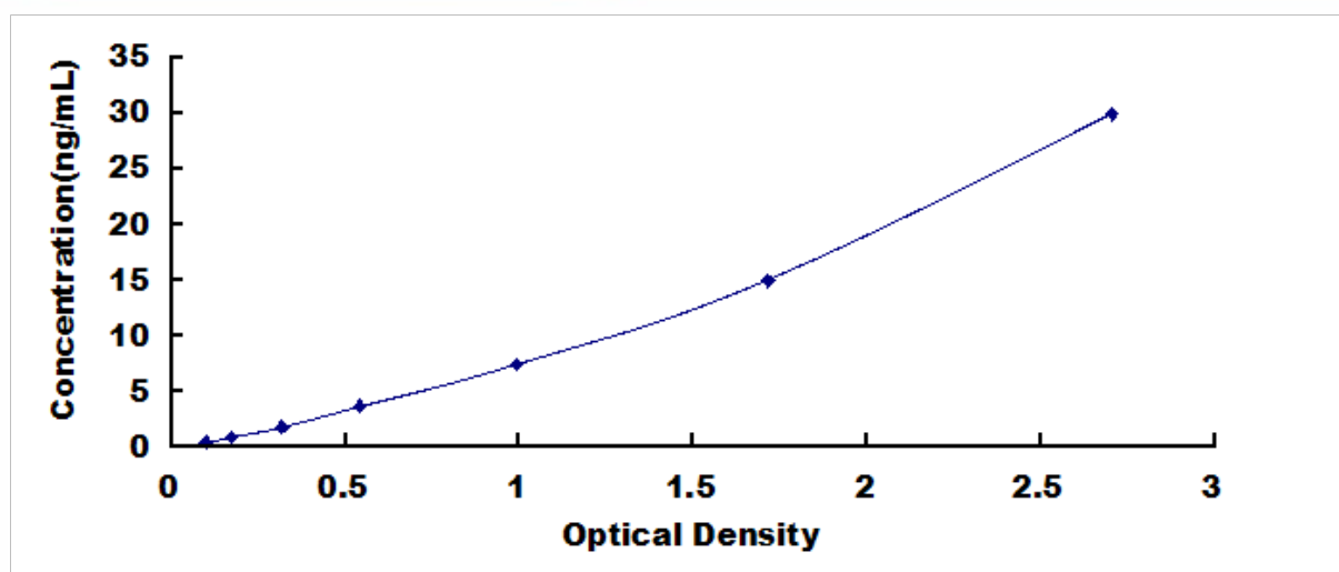
人尿胰蛋白酶抑制剂 (UTI) 检测试剂盒标准曲线
