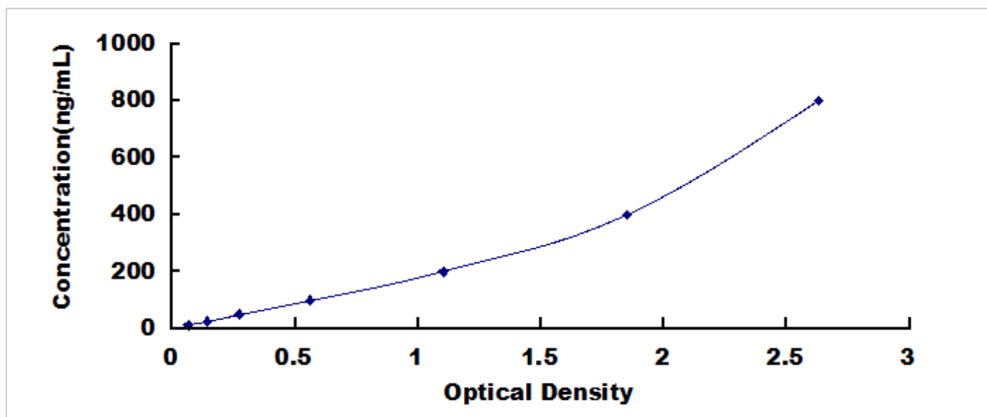
人尿调蛋白 (UMOD) 检测试剂盒标准曲线
