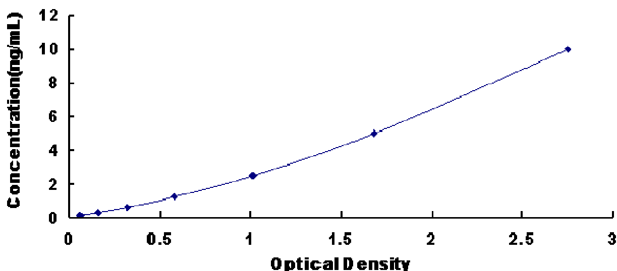
人 V-Re1 网状内皮增生病毒癌基因同源物 B (RELB) 试剂盒标准曲线
