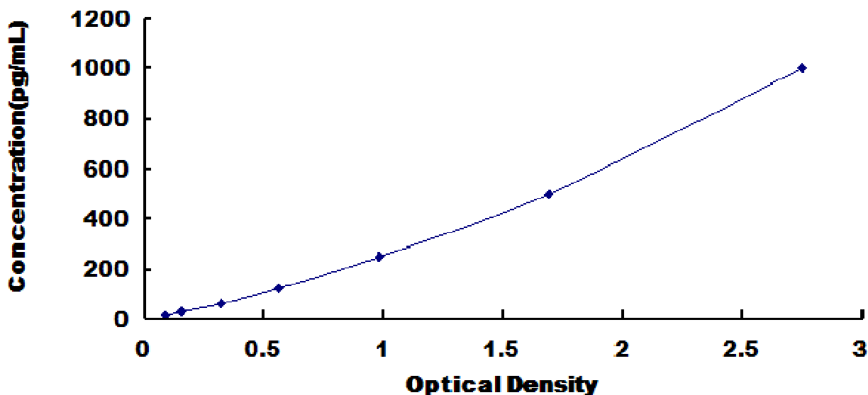
人血管内皮生长因子 121 (VEGF121) 检测试剂盒标准曲线
