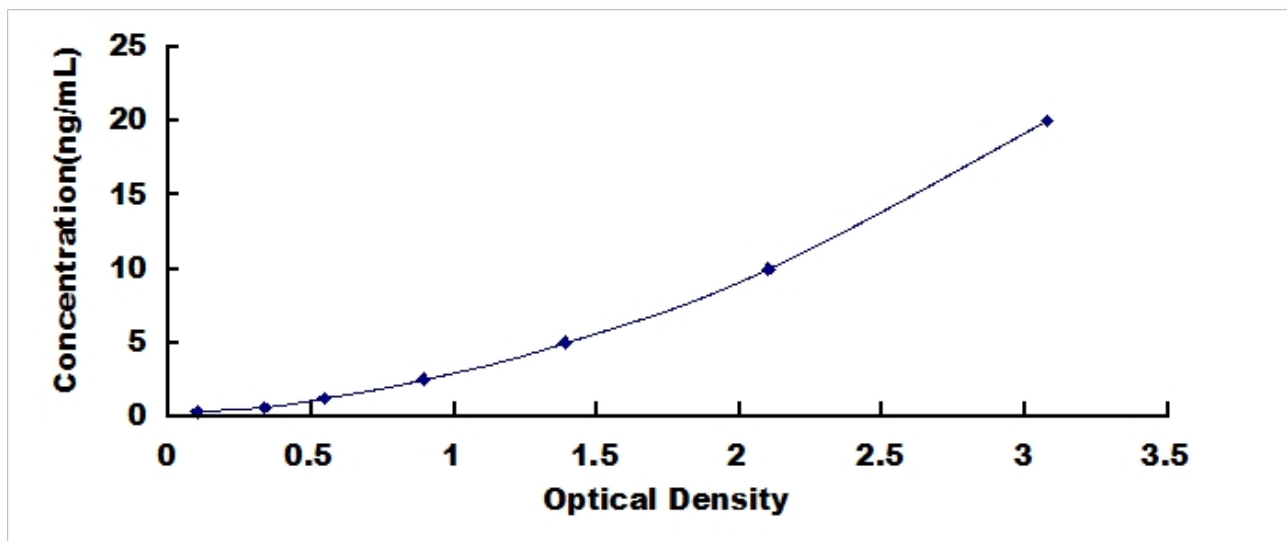
小鼠波形蛋白 (VIM) 检测试剂盒标准曲线
