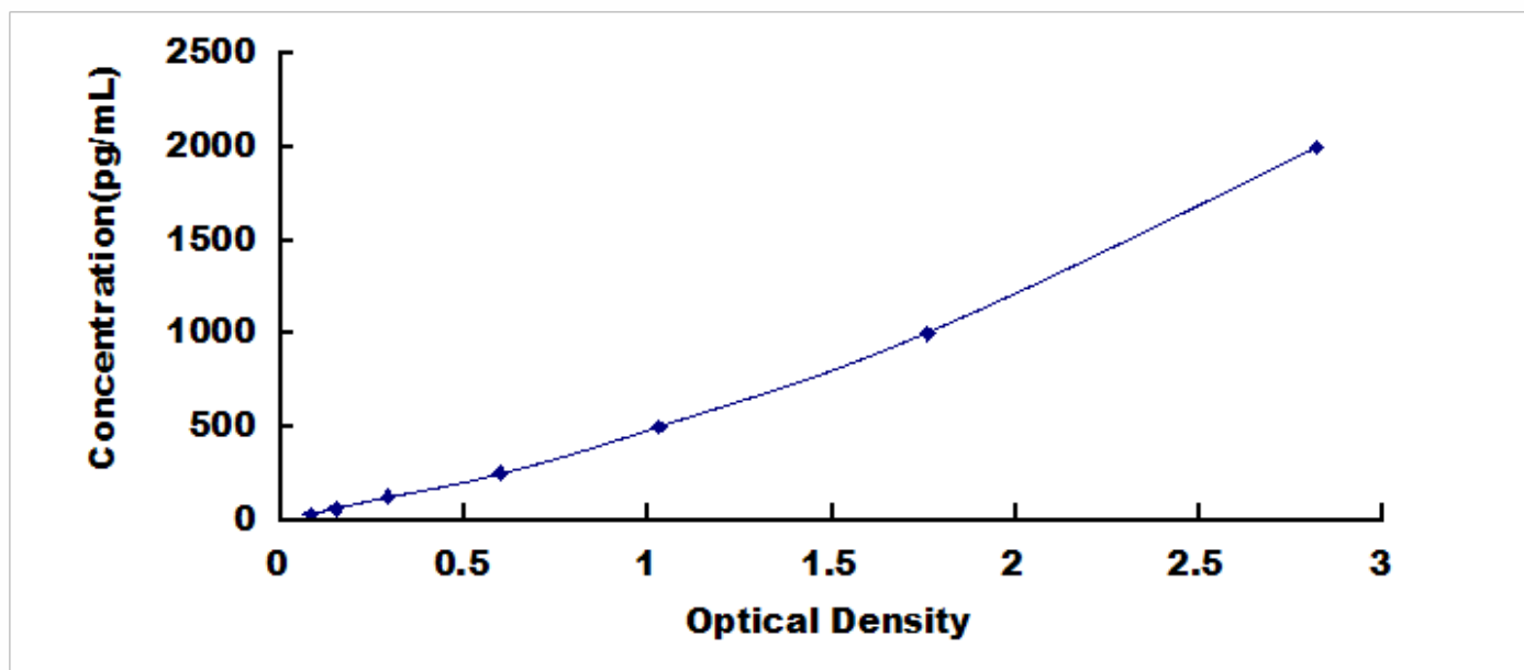
小鼠内脂素(VF)检测试剂盒标准曲线
