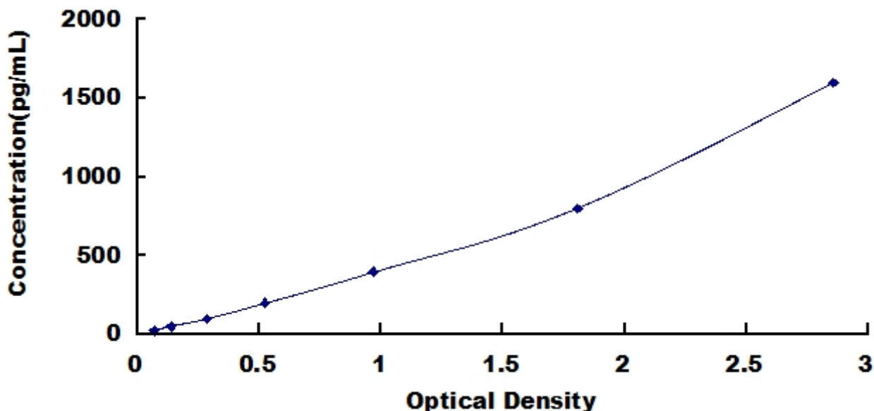
小鼠血管性血友病因子(vWF)检测试剂盒标准曲线
