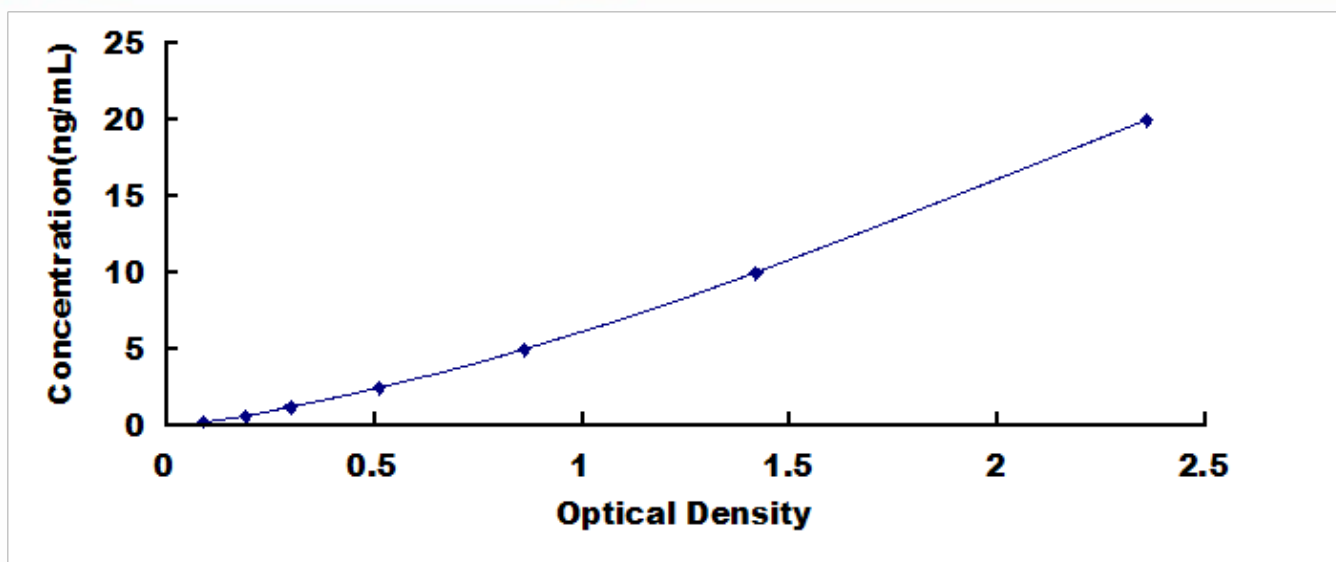
人 WAP 四二硫化物核心域蛋白 2 (WFDC2) 检测试剂盒标准曲线
