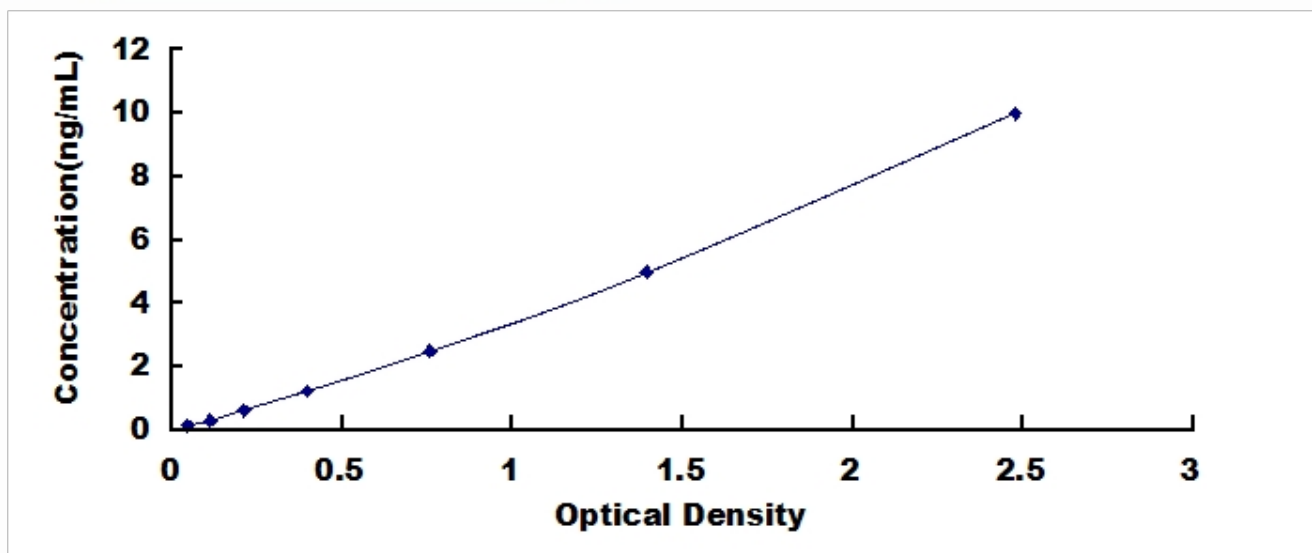
人淀粉酶 \alpha (Amya) 检测试剂盒标准曲线
