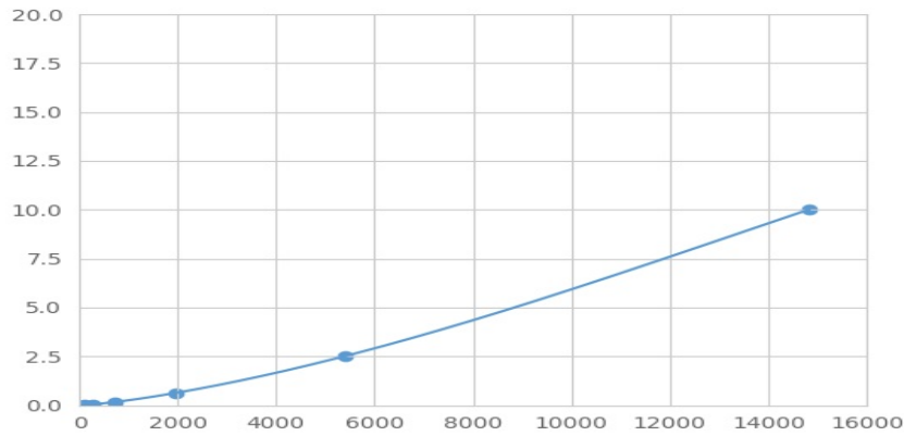
(钙离子转运ATP酶A2)检测试剂盒标准曲线
