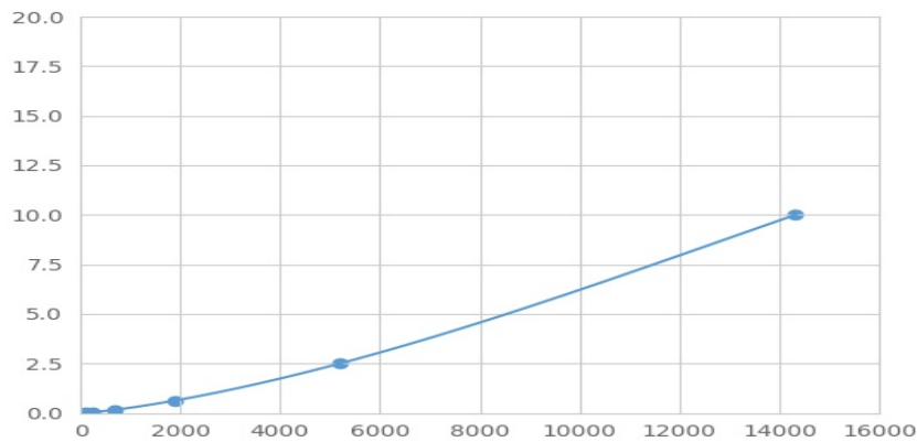
(氢离子转运ATP酶线粒体F1复合体β肽)检测试剂盒标准曲线
