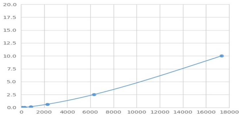
(芳香烃受体核转位因子样蛋白)检测试剂盒标准曲线
