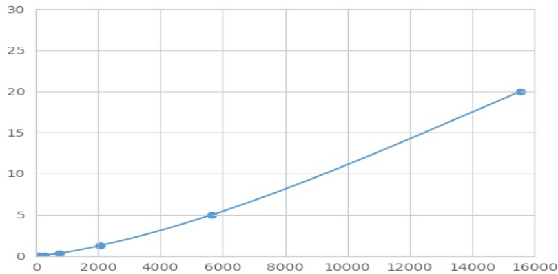
(脆性X智力迟钝蛋白1)检测试剂盒标准曲线
