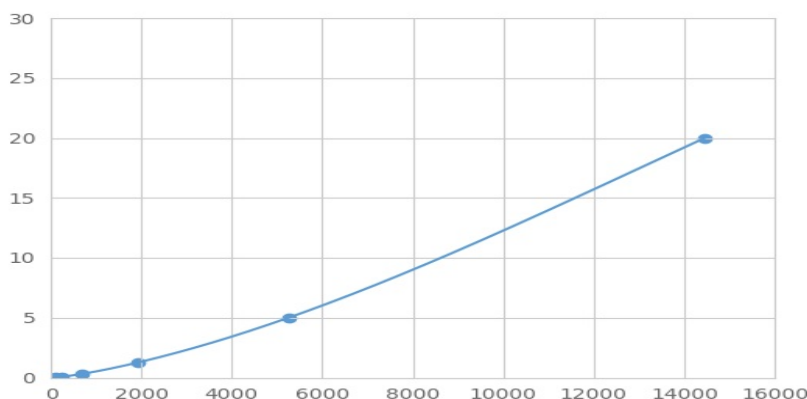
(卷曲同源物6)检测试剂盒标准曲线
