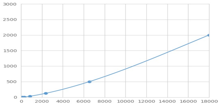
(角蛋白6C)检测试剂盒标准曲线
