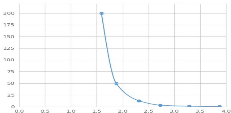
(犬尿酸)检测试剂盒标准曲线
