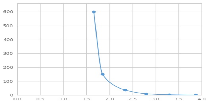
(乳酸)检测试剂盒标准曲线
