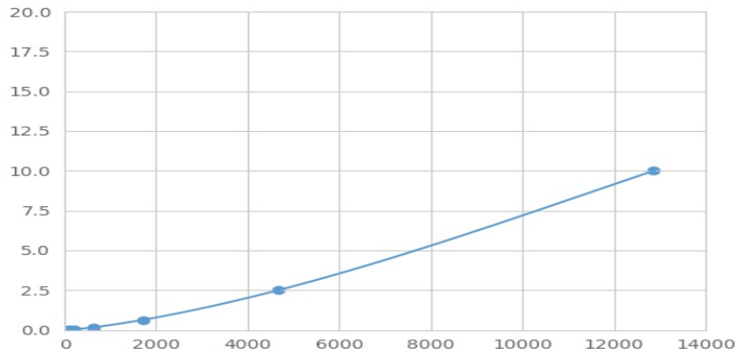
(黑色素瘤抗原家族B16)检测试剂盒标准曲线
