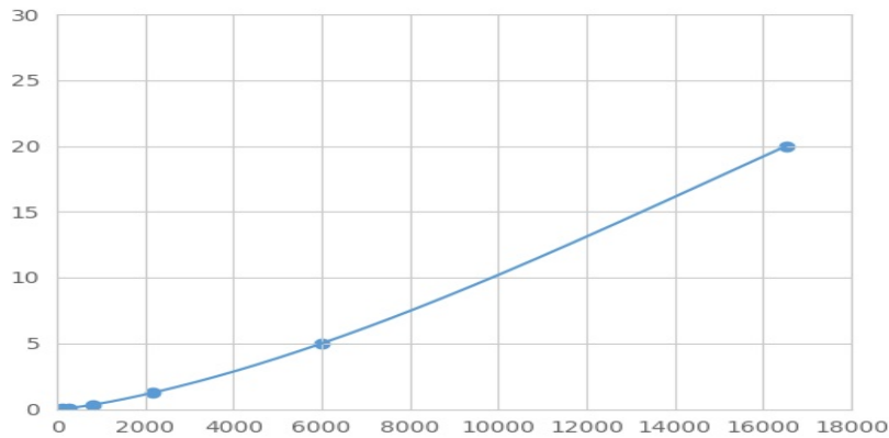
(磷酸酶张力蛋白同源物)检测试剂盒标准曲线
