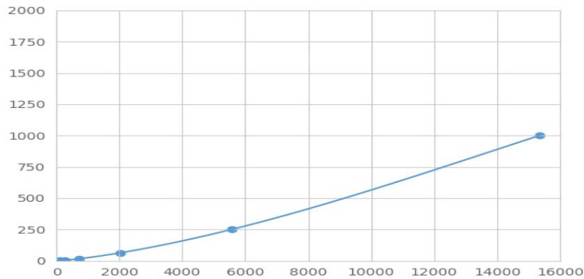
(尿激酶型纤溶酶原激活因子)检测试剂盒标准曲线
