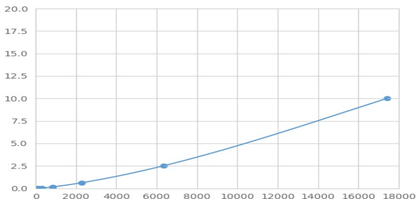
(Rac-GTP酶激活蛋白1)检测试剂盒标准曲线
