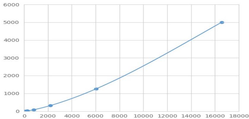
(肿瘤蛋白p53诱导蛋白3)检测试剂盒标准曲线
