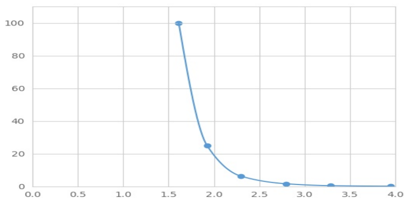
(酪氨酸)检测试剂盒标准曲线
