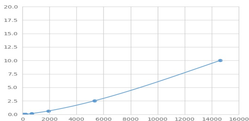
(V-Ets骨髓成红细胞增多症病毒E26癌基因同源物1)检测试剂盒标准曲线
