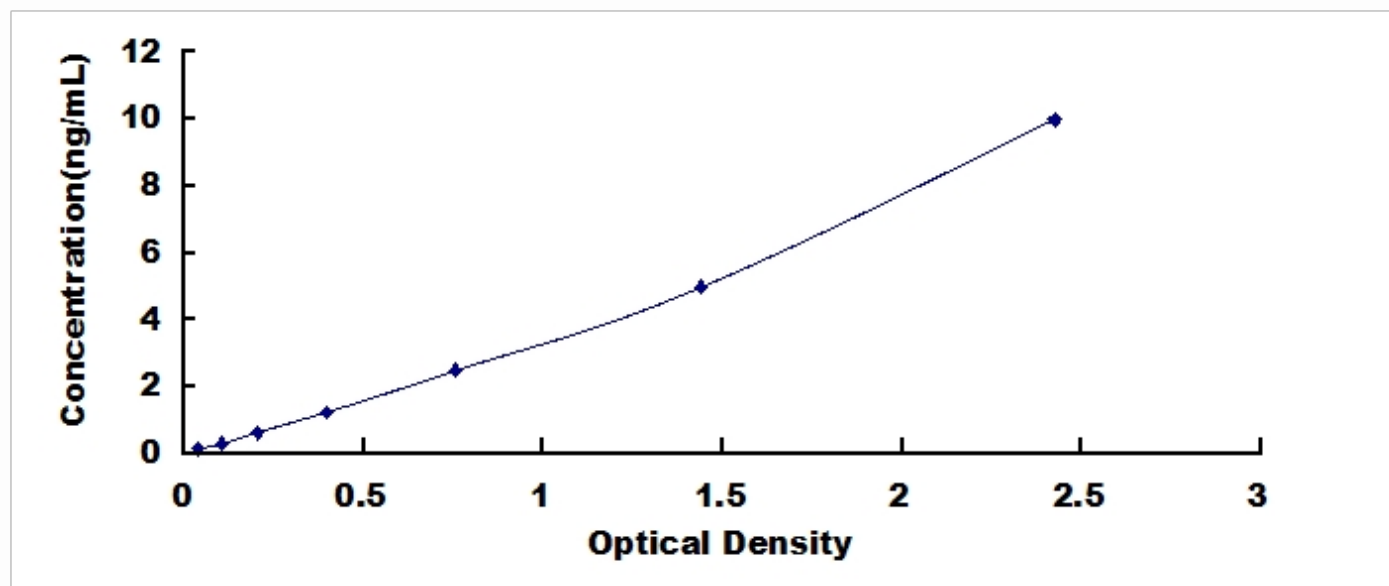
小鼠血小板衍生生长因子 BB (PDGFBB) 检测试剂盒标准曲线
