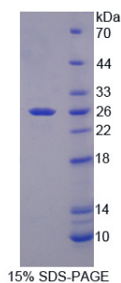
15% SDS-PAGE
